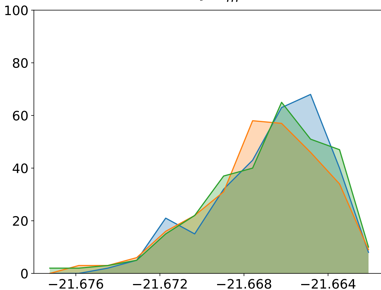
(e) J(x_c^*)
