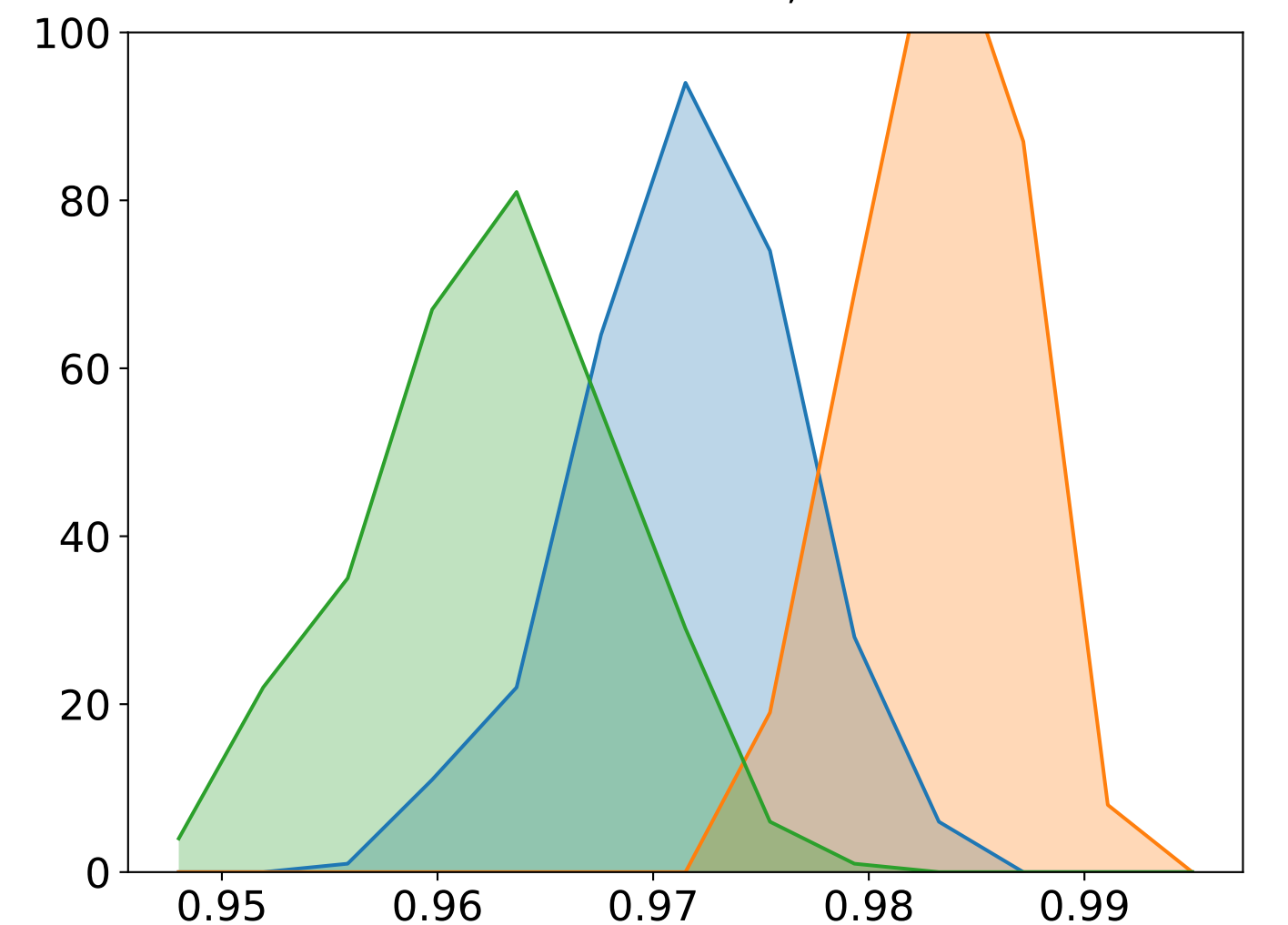
(f) CEC_{0,l',z}
