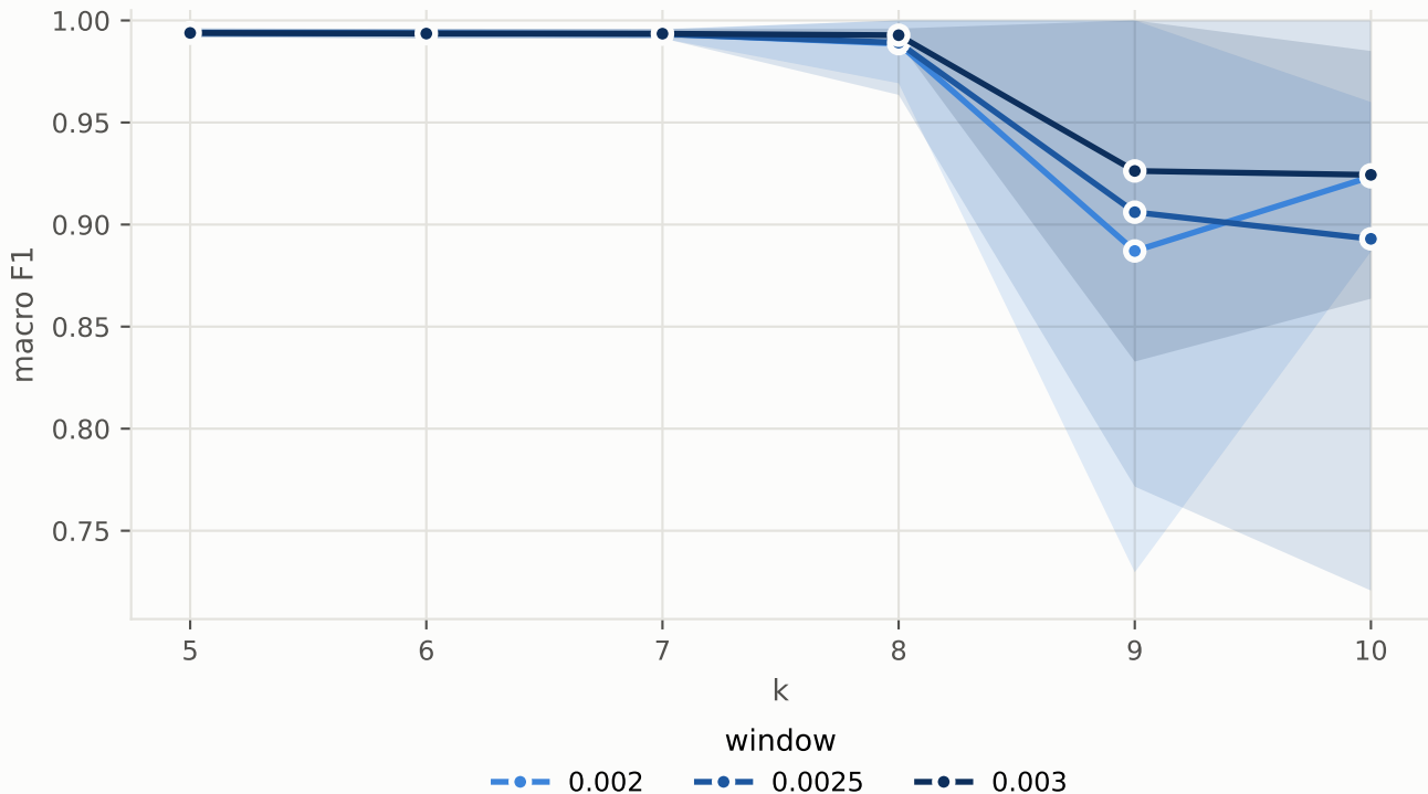
GREAC · denv — macro F1 × k per window (mean ± 1 SD)
