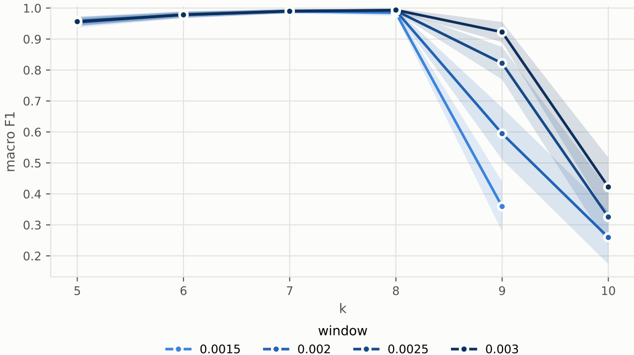
GREAC · hiv — macro F1 × k per window (mean ± 1 SD)
