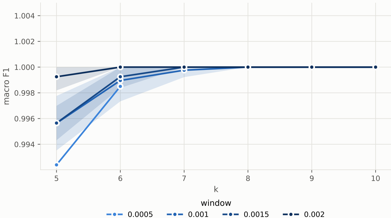
GREAC · mkpx — macro F1 × k per window (mean ± 1 SD)
