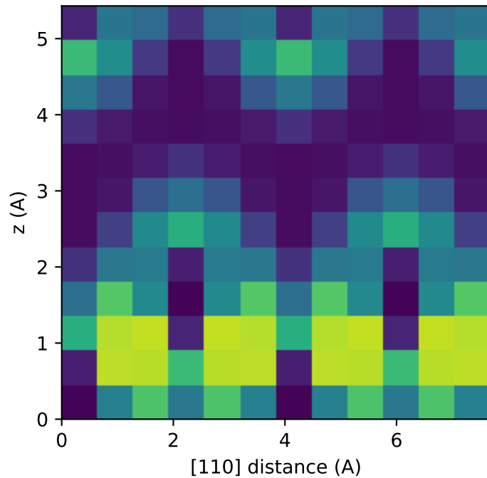
Strong: 1.548 fs
