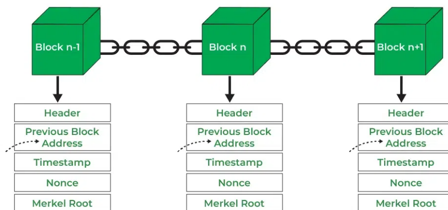
شکل ۲: ساختار عمومی زنجیره بلوکی: زنجیره‌ای از بلوک‌ها با اتصال هش هر بلوک به بلوک قبلی
