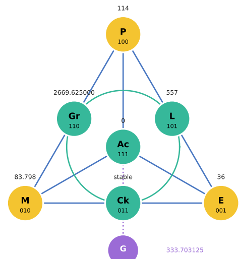
36 Kr • Krypton
