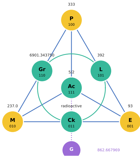
93 Np · Neptunium
