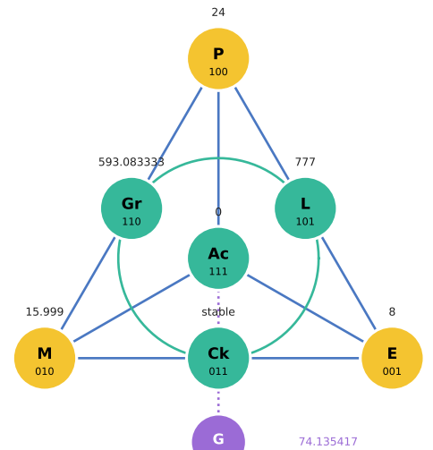
12 Mg · Magnesium
