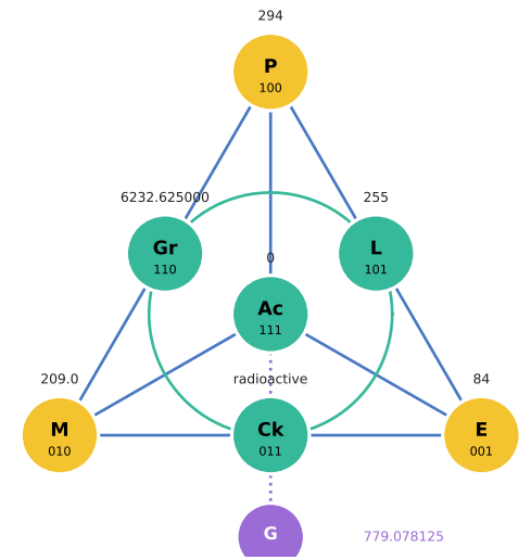
84 Po · Polonium
