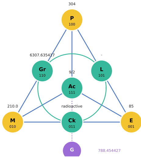
89 Ac · Actinium
