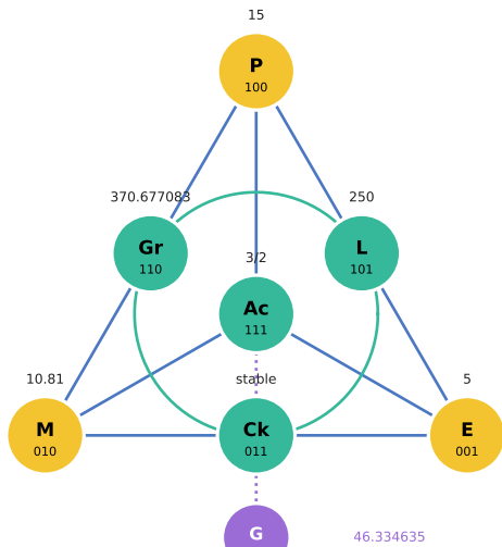
9 F · Fluorine
