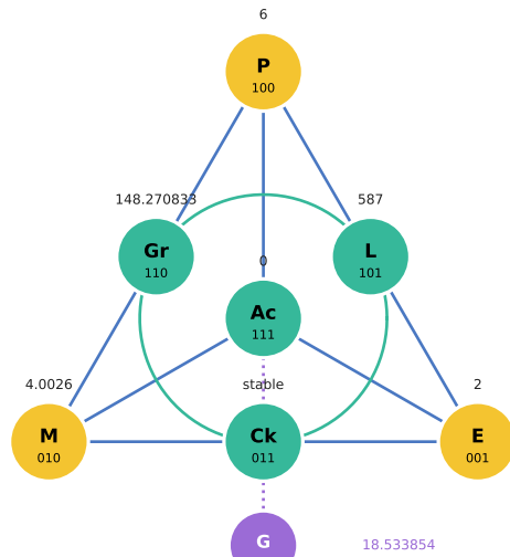
6 C · Carbon
