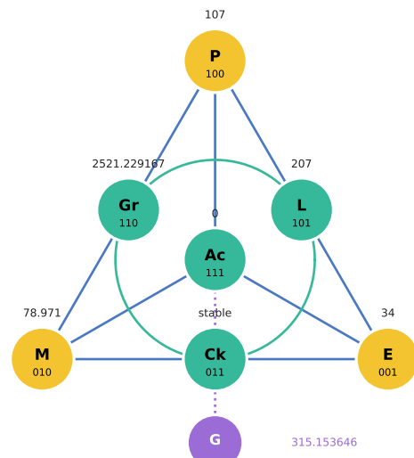
34 Se • Selenium
