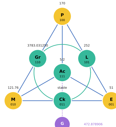
55 Cs · Caesium
