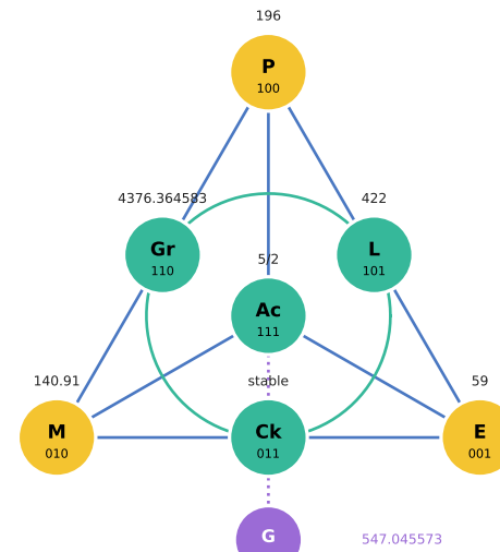
59 Pr · Praseodymium
