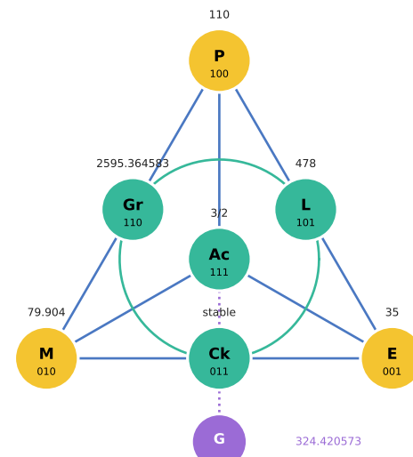
35 Br • Bromine
