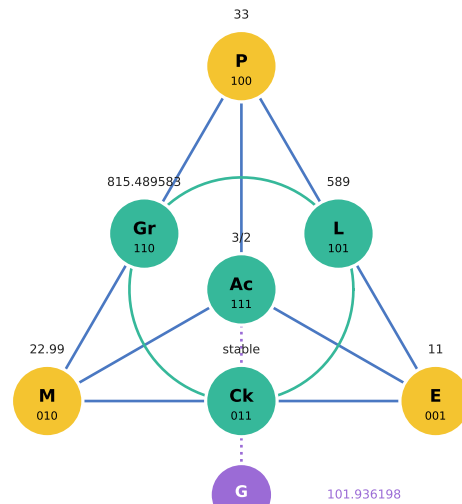
11 Na · Sodium
