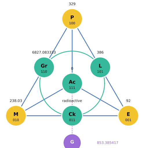
96 Cm · Curium
