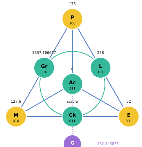
56 Ba · Barium
