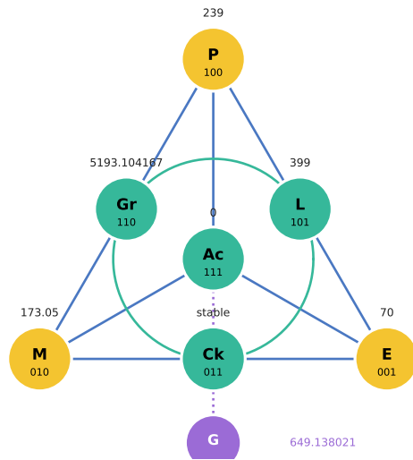
70 Yb · Ytterbium
