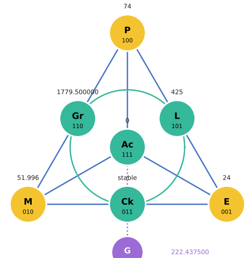
24 Cr · Chromium
