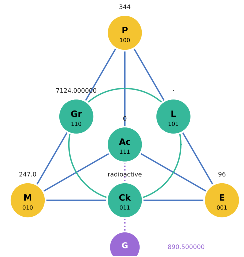
96 Cm · Curium
