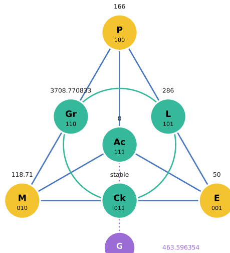
54 Xe · Xenon
