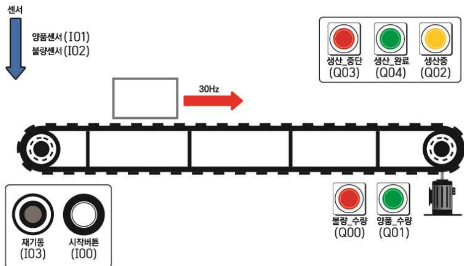
[구성도]
