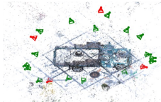
ACP
