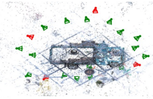
Ours
