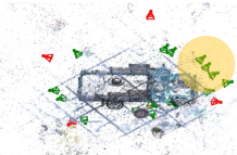
MUSIQ
