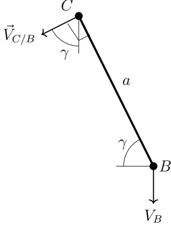
Figura 5: Diagrama de velocidad relativa \vec{V}_{C/B} respecto al brazo CB .
