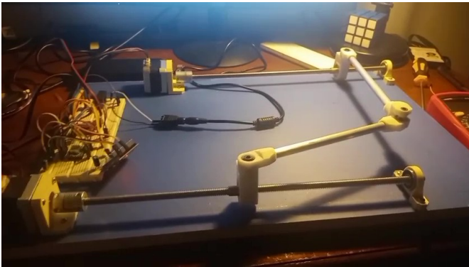
Figura 6: Montaje mecánico del prototipo
