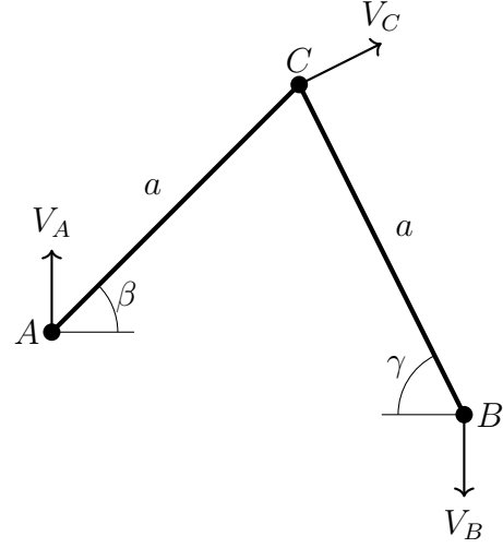
Figura 3: Diagrama cinemático del problema.
