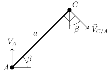
Figura 4: Diagrama de velocidad relativa \vec{V}_{C/A} respecto al brazo AC.
