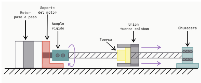
Figura 2: Alternativa tornillo-tuerca
