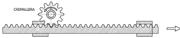
Figura 1: Alternativa piñon-cremallera
