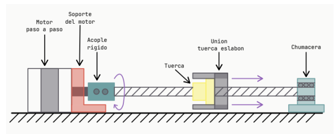
Figura 2: Alternativa tornillo-tuerca
