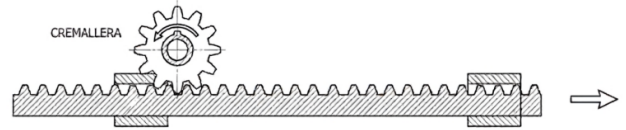
Figura 1: Alternativa piñón-cremallera
