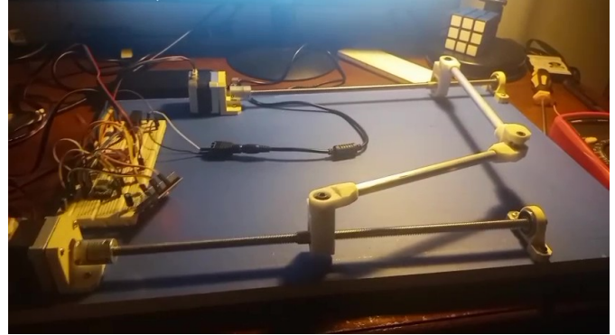
Figura 3: Montaje mecánico del prototipo
