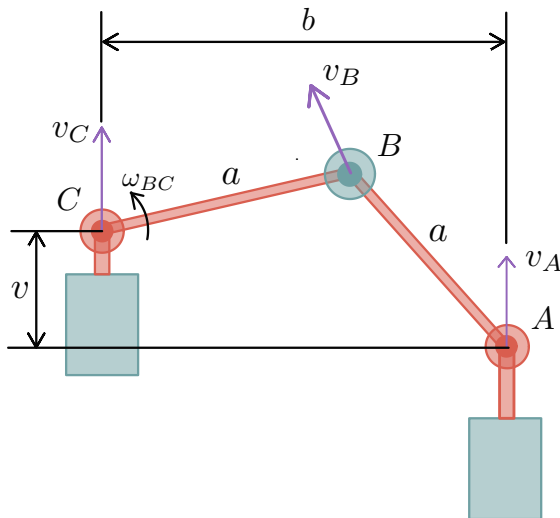
Figura 1: Mecanismo planteado.
