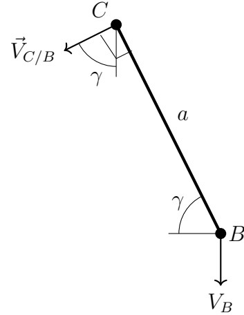
Figura 9: Diagrama de velocidad relativa \vec{V}_{C/B} respecto al brazo CB .
