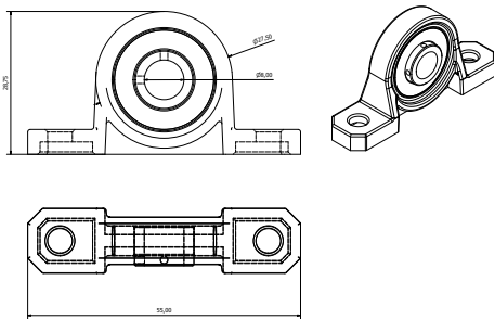
Figura 15: Chumacera.
