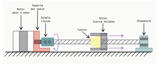
Figura 3: Alternativa tornillo-tuerca
