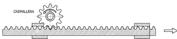
Figura 2: Alternativa piñón-cremallera
