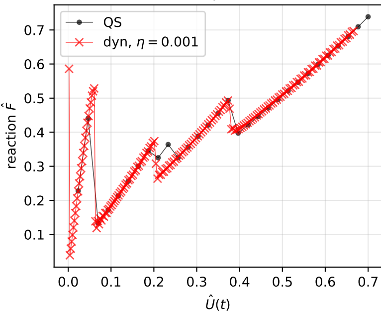
Force-displacement
