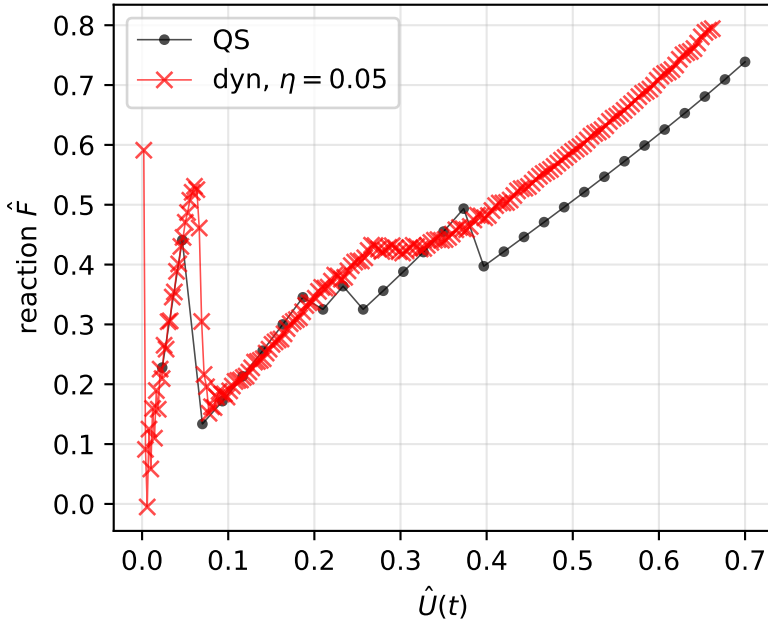
Force-displacement
