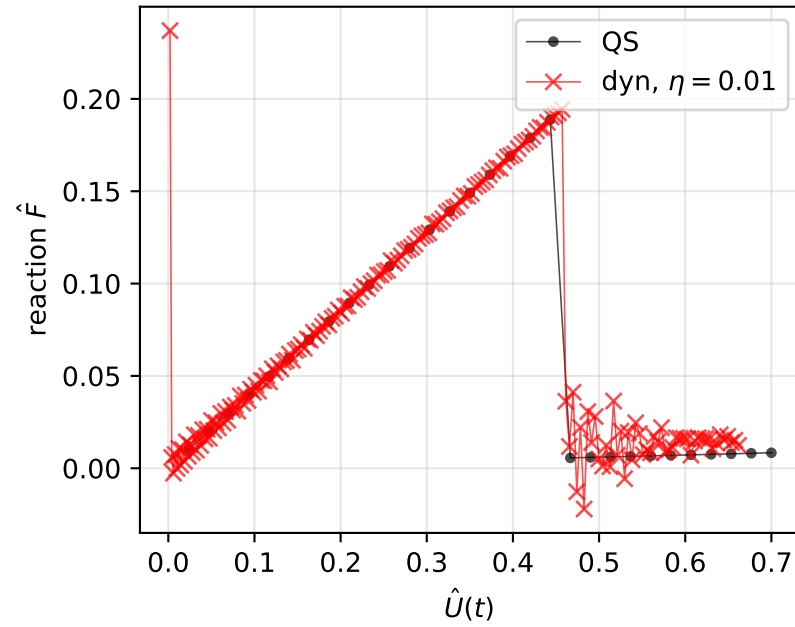
Force-displacement
