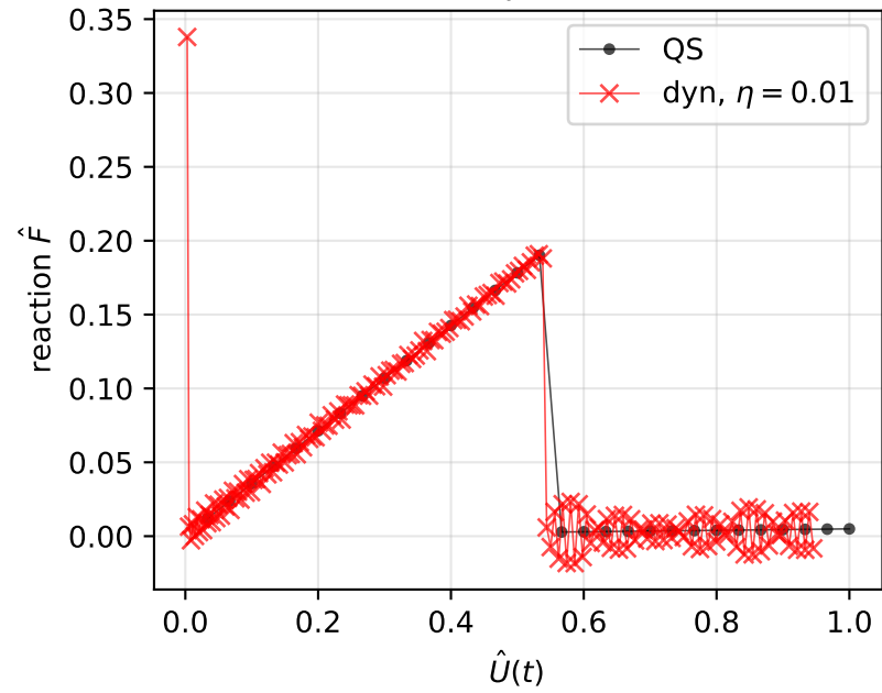
Force-displacement
