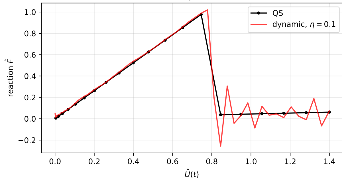
Force-displacement
