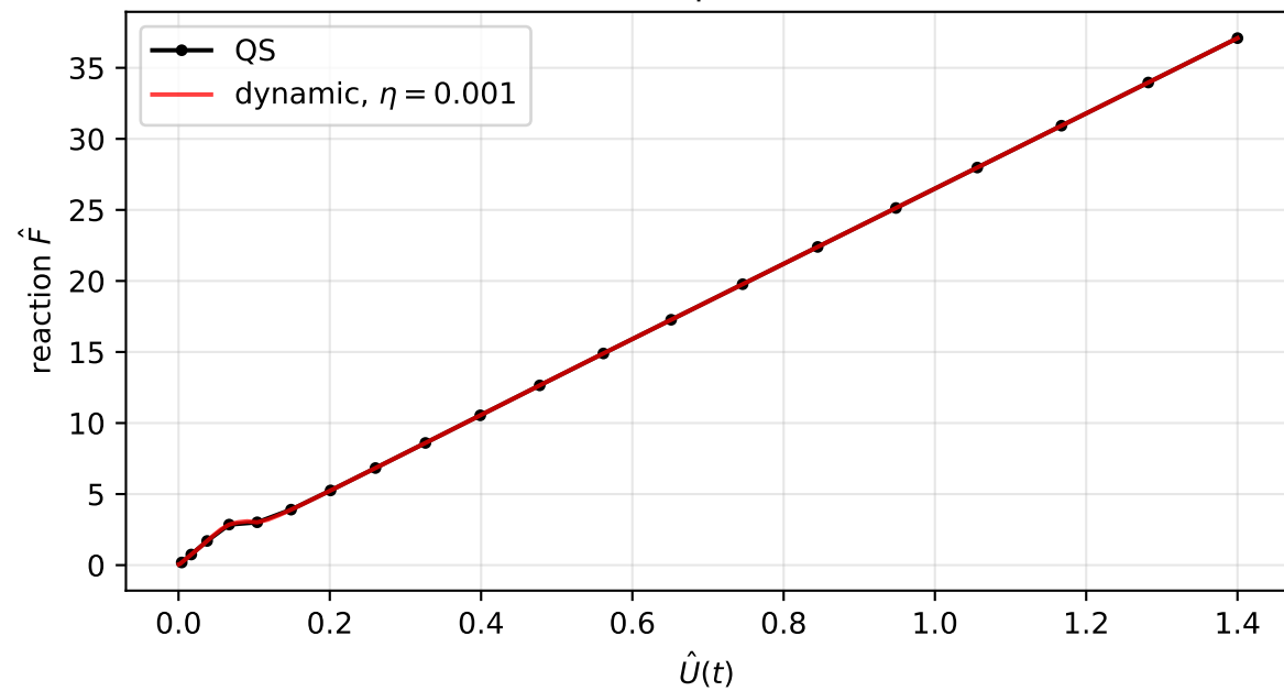
Force-displacement
