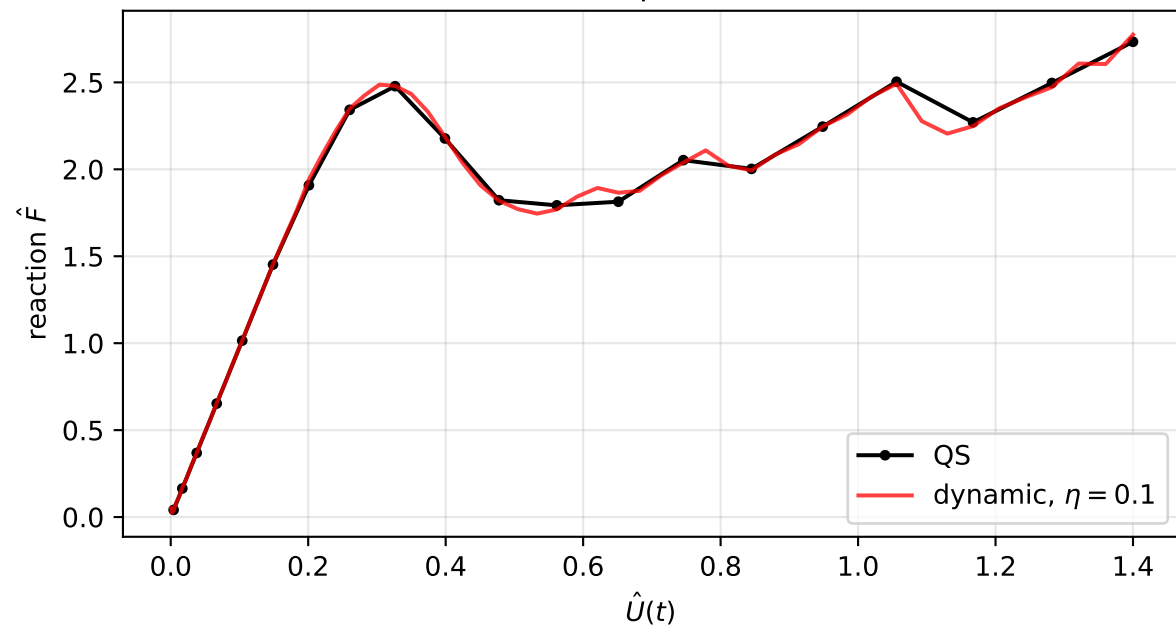
Force-displacement
