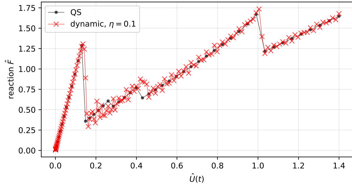
Force-displacement
