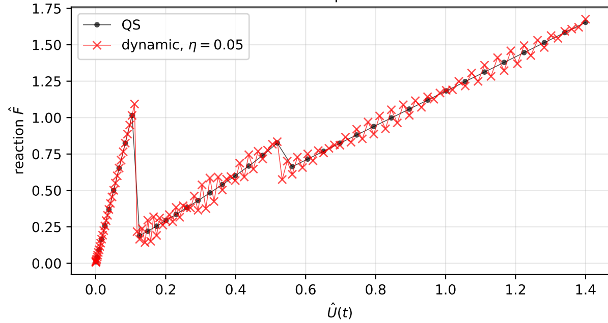
Force-displacement
