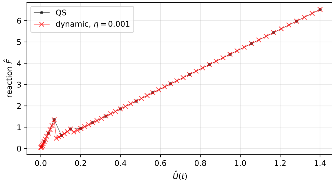
Force-displacement
