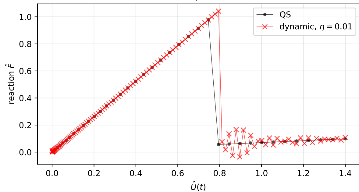
Force-displacement
