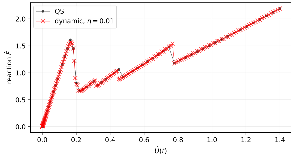
Force-displacement
