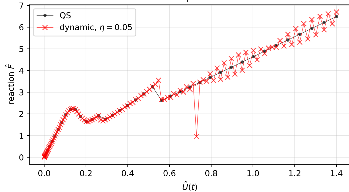
Force-displacement
