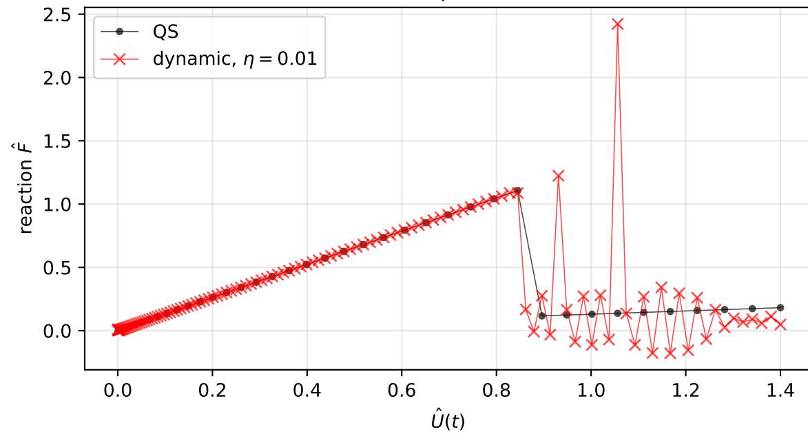
Force-displacement
