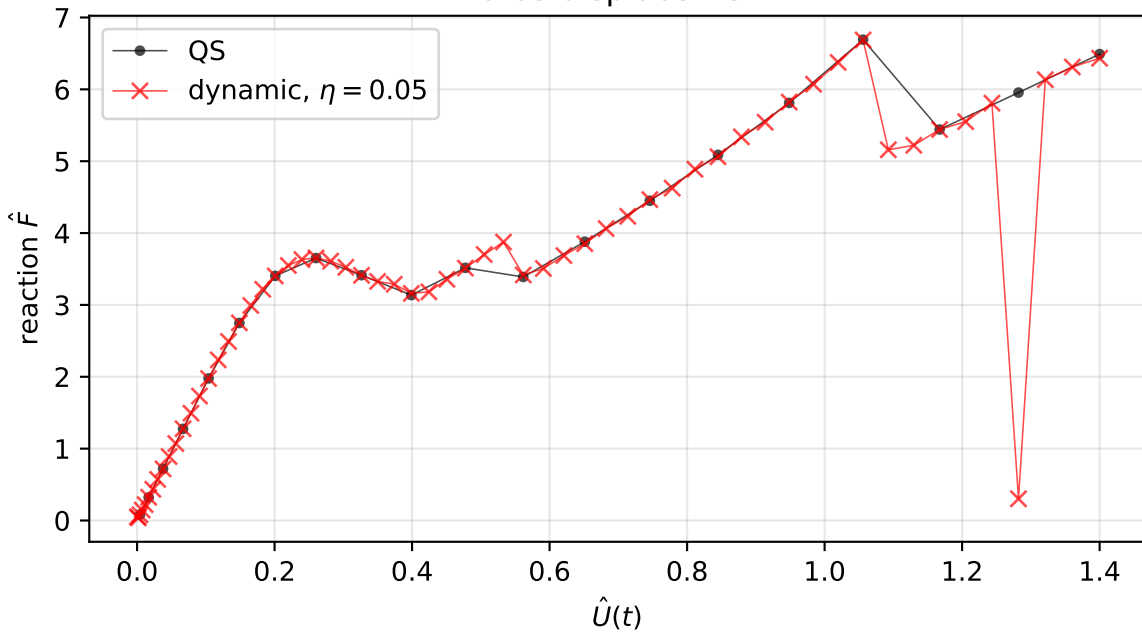
Force-displacement
