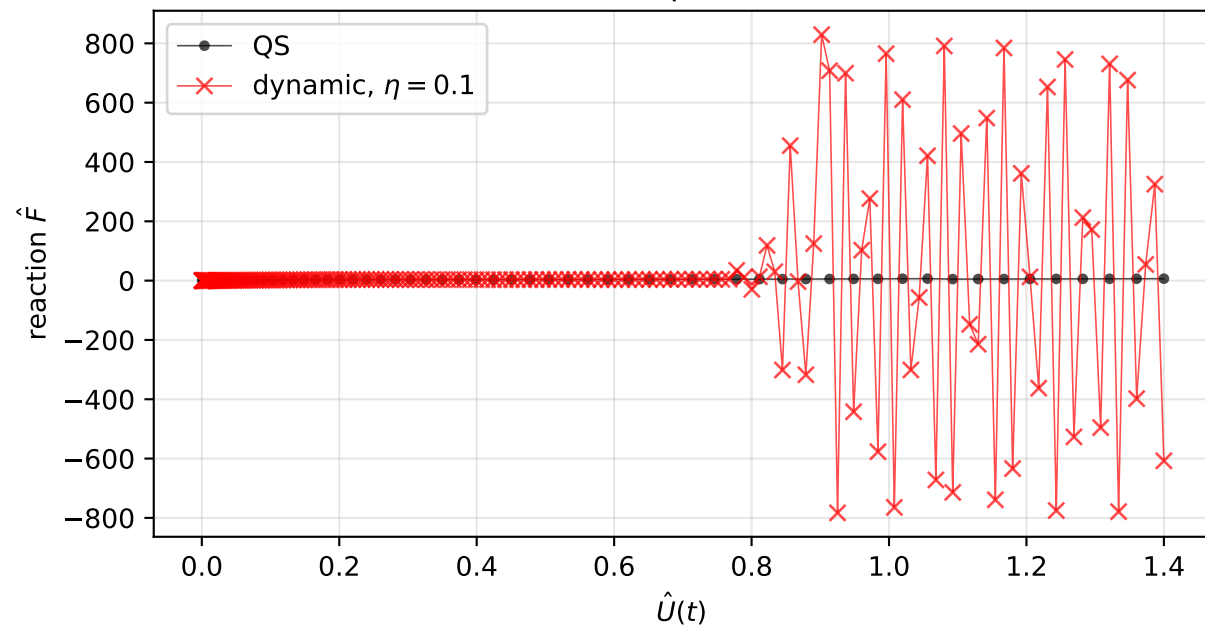
Force-displacement
