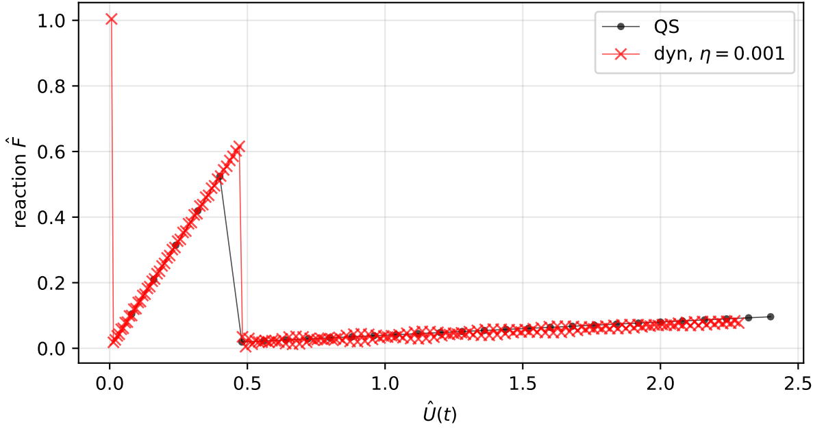
Force-displacement
