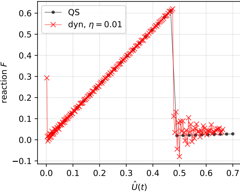
Force-displacement
