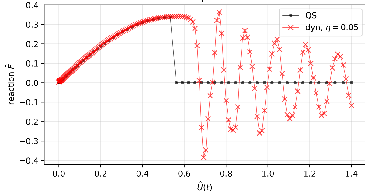
Force-displacement
