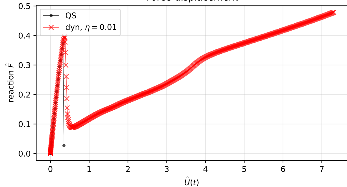
Force-displacement
