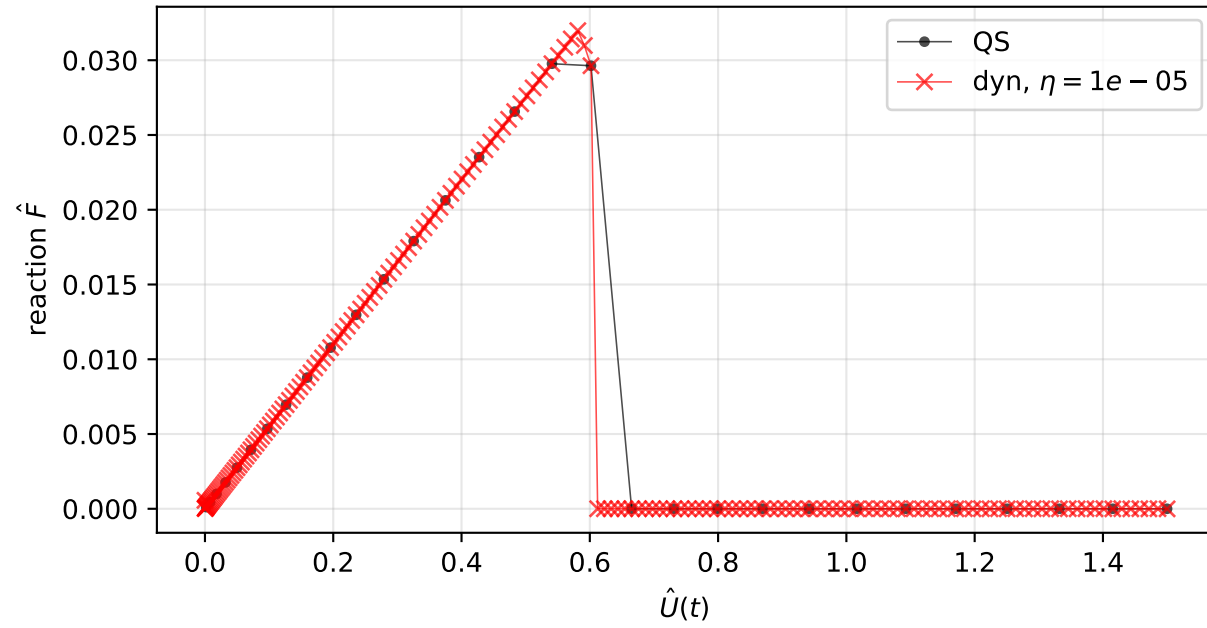
Force-displacement
