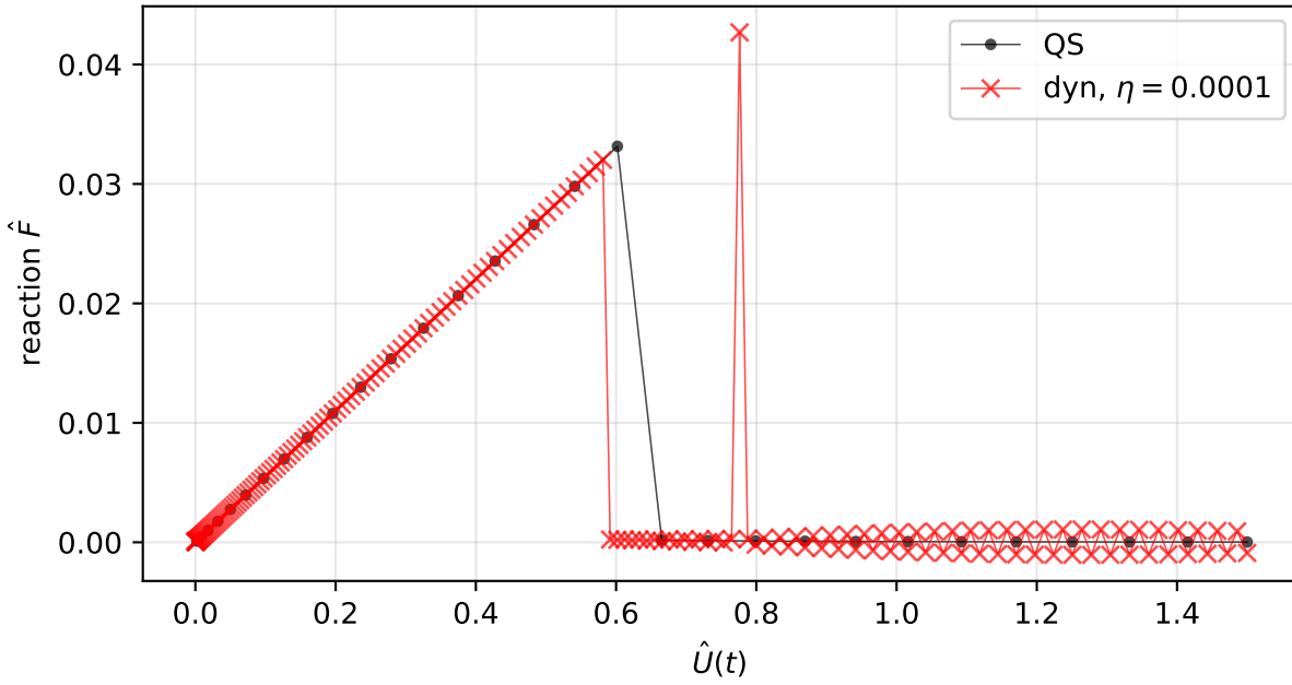
Force-displacement
