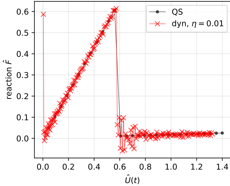
Force-displacement
