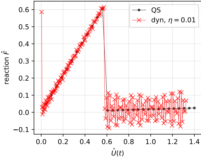
Force-displacement
