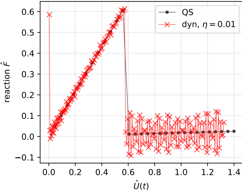
Force-displacement
