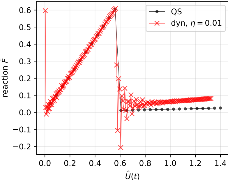
Force-displacement
