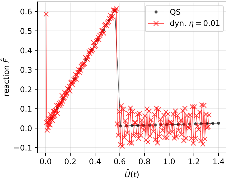
Force-displacement
