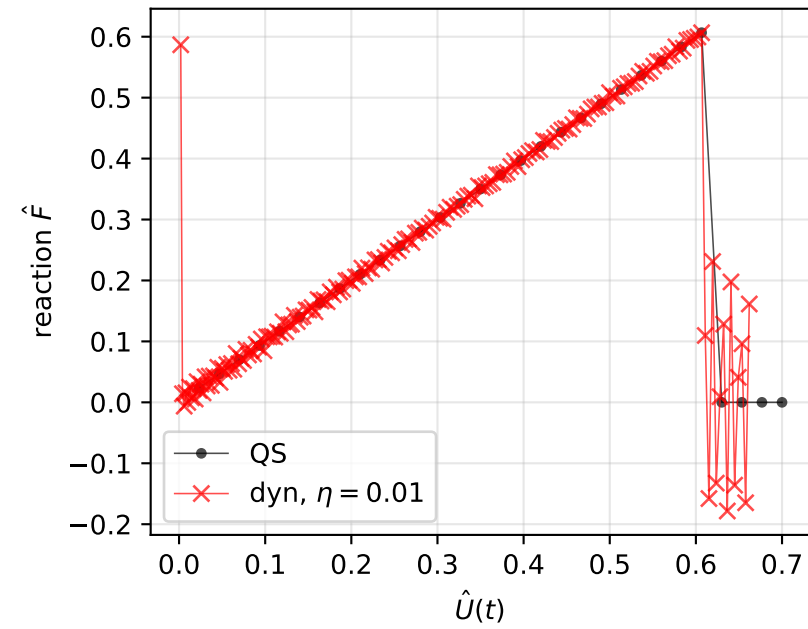
Force-displacement
