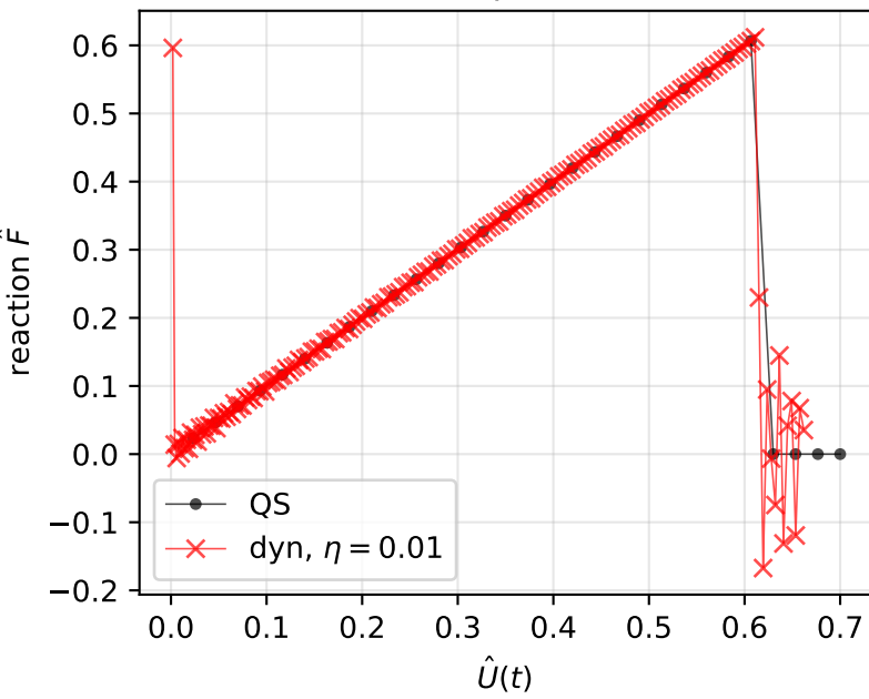
Force-displacement
