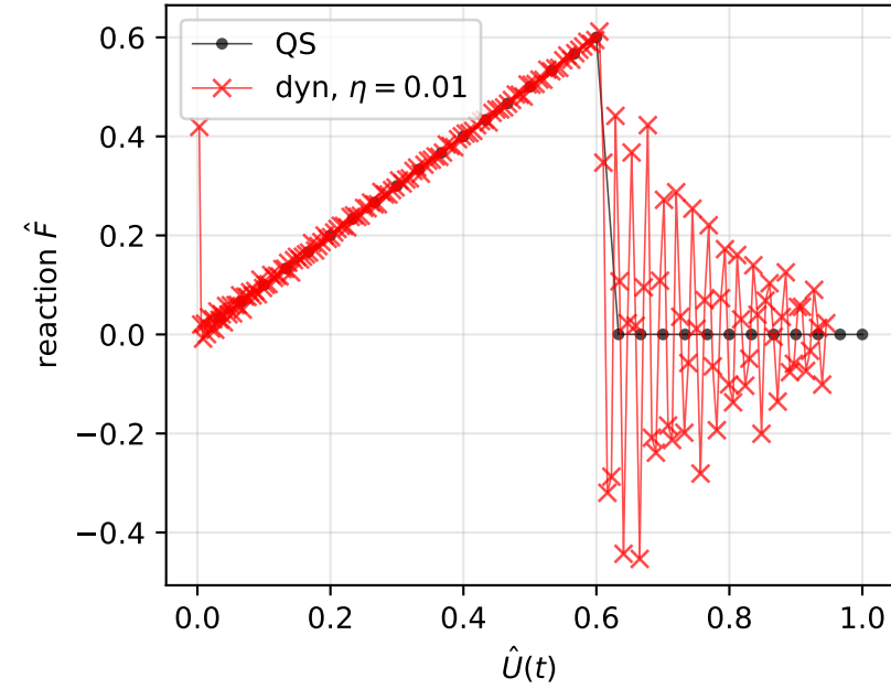
Force-displacement
