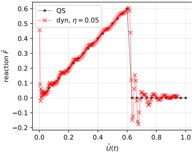
Force-displacement
