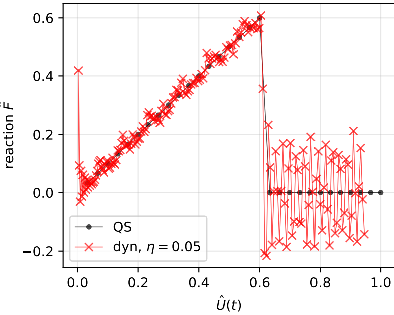
Force-displacement
