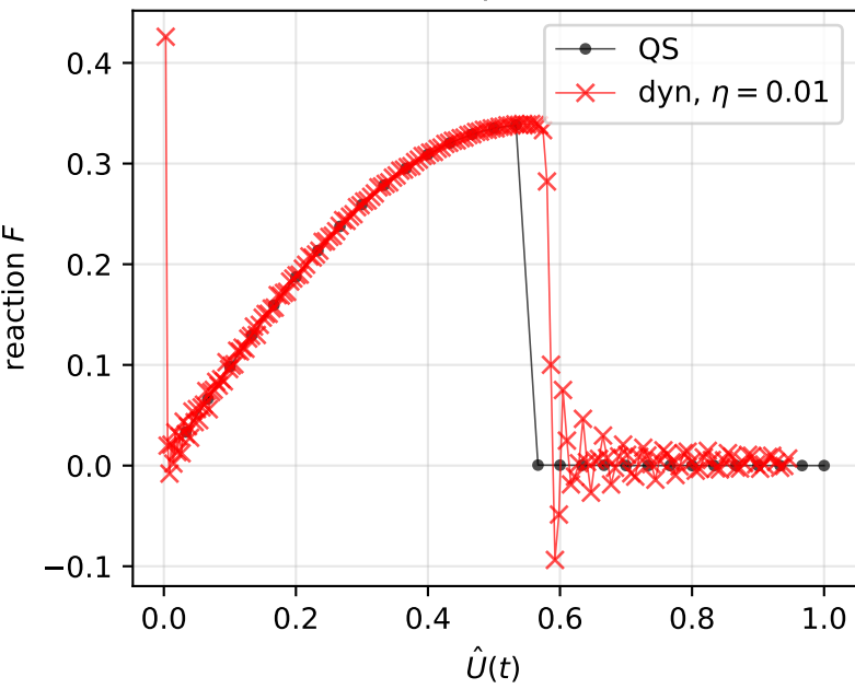
Force-displacement
