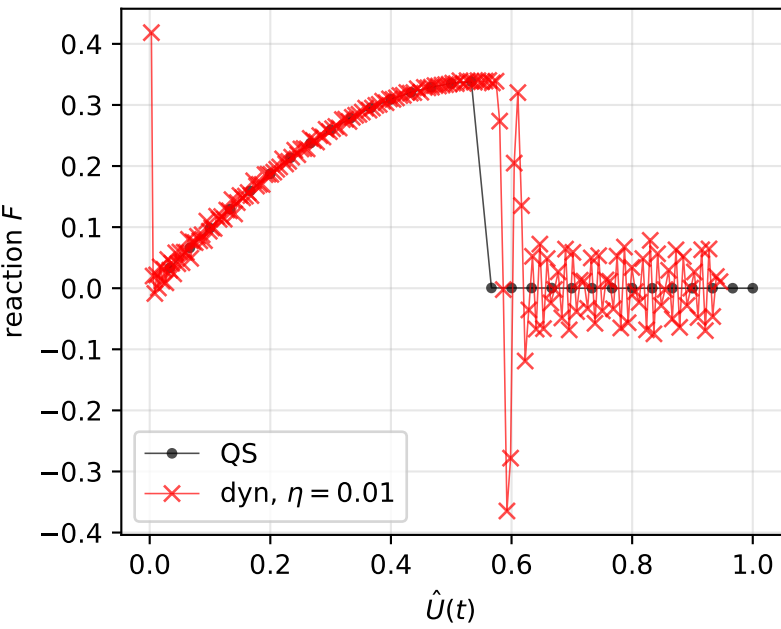
Force-displacement
