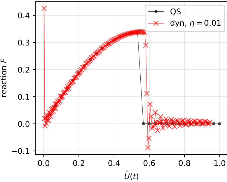
Force-displacement
