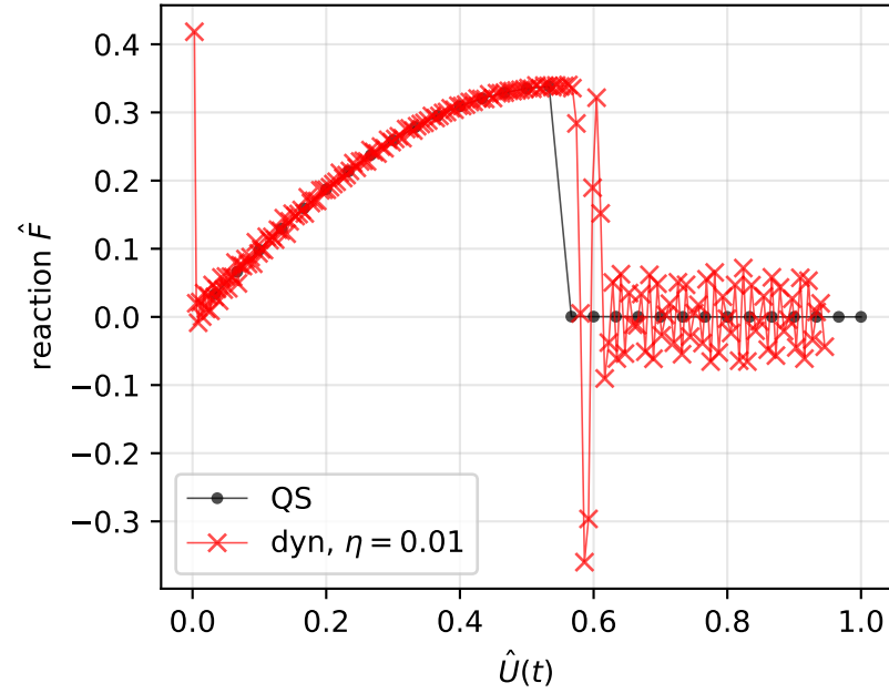
Force-displacement
