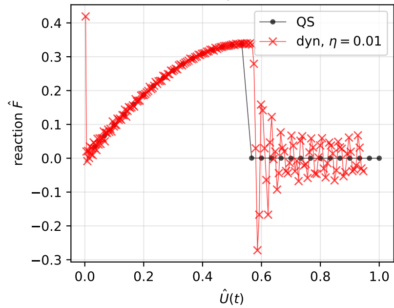
Force-displacement
