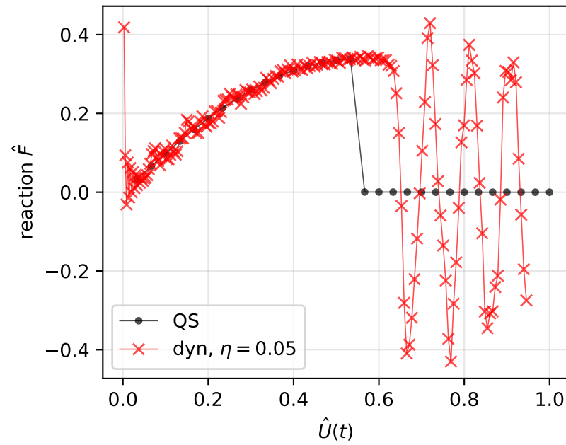
Force-displacement
